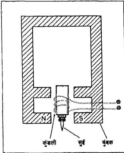
चित्र 19 विद्युत चुंबक पिक-अप
