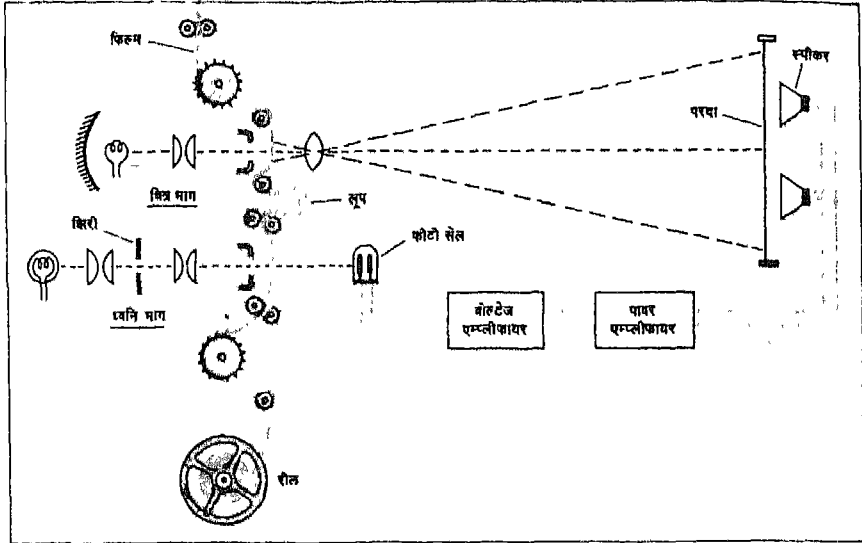
चित्र 31 फिल्म पर अंकित ध्वनि का प्तरूपादन
